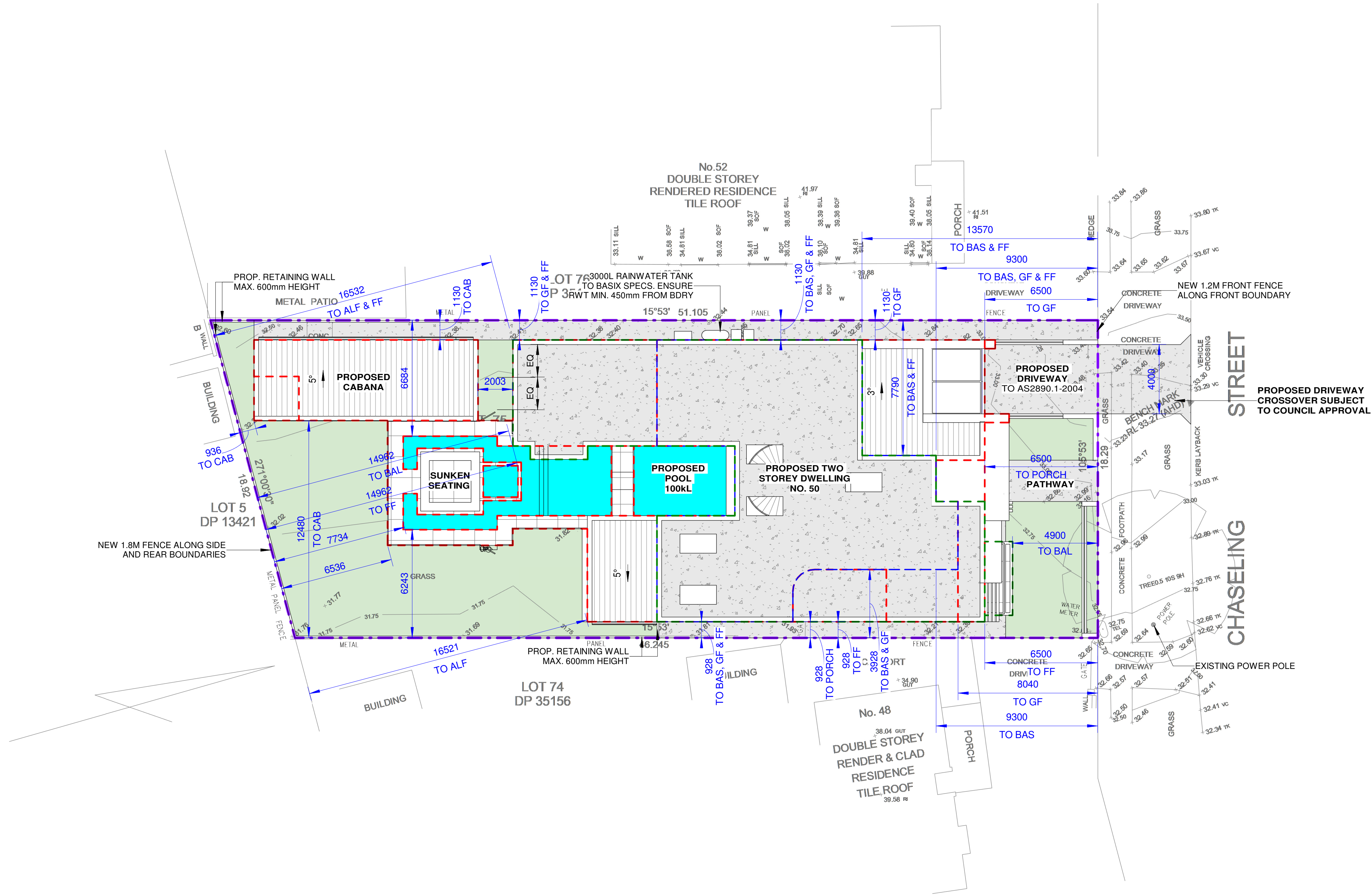
1 SITE PLAN & ROOF PLAN, SITE ANALYSIS PLAN 1 : 200
